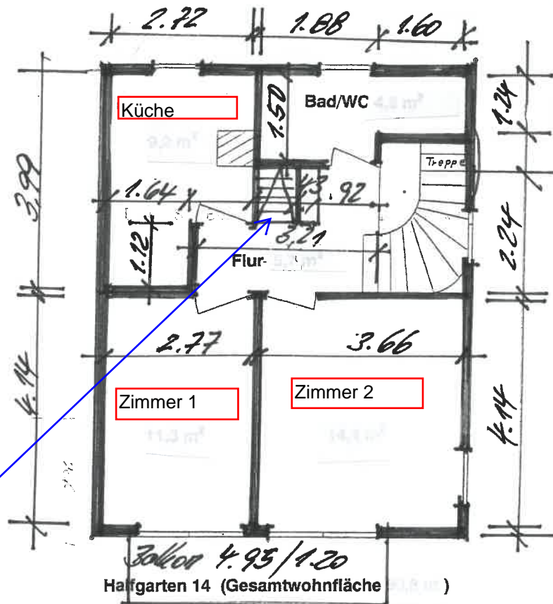
Plan Dachgeschoss
