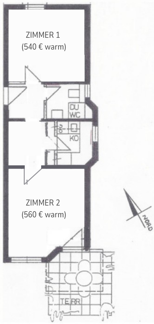
Grundriss
